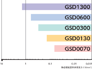
额定承重图
