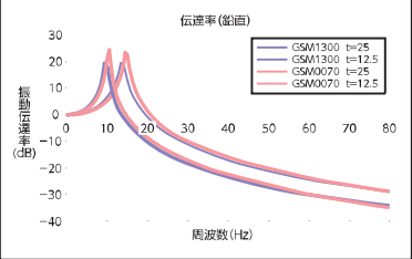
传递特性图
